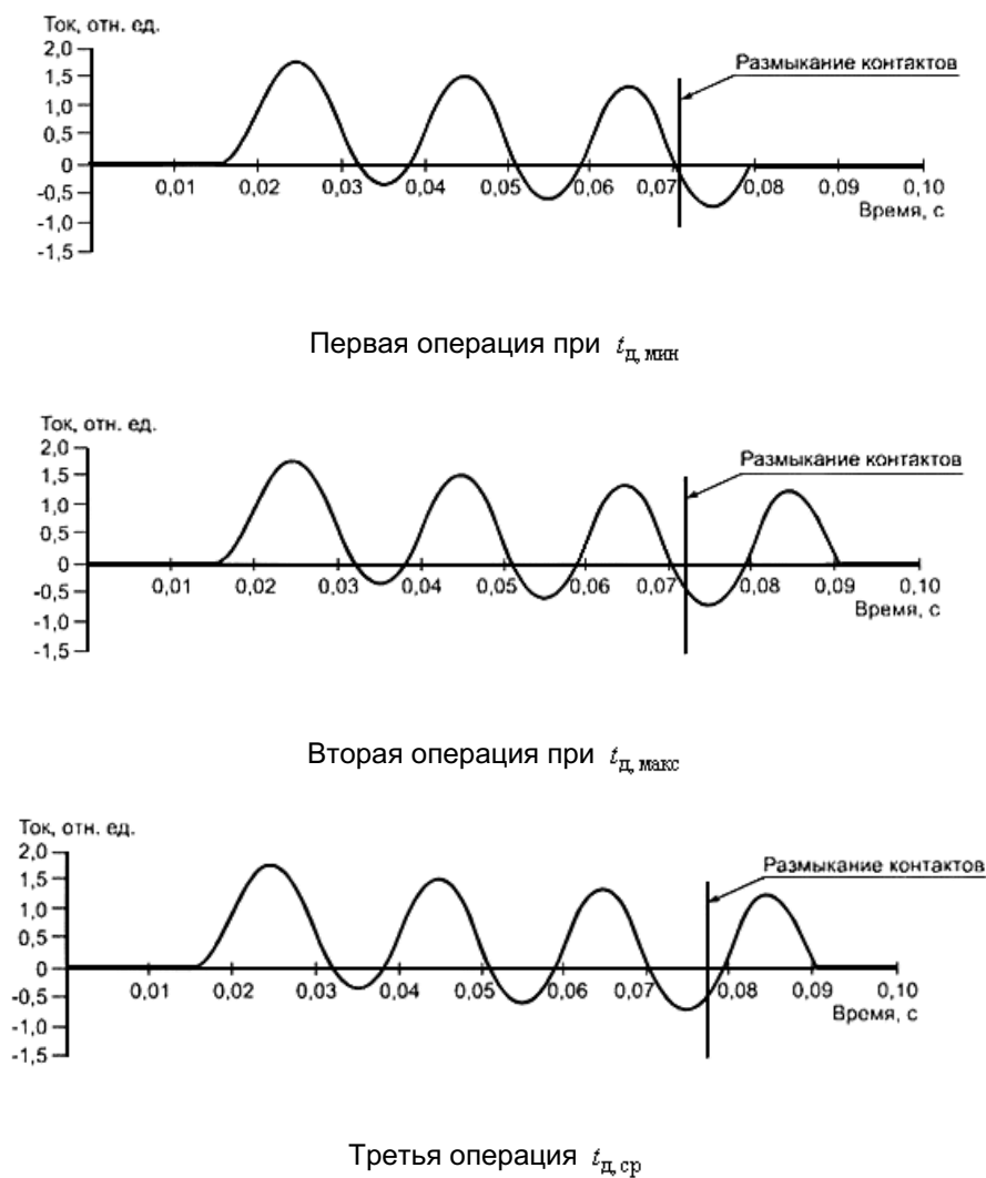
Рисунок 14 - Регулирование моментов инициирования тока и размыкания контактов при однополюсном отключении тока в режиме Т100а выключателями с U_{\text{ном}} \geq 110 кВ
